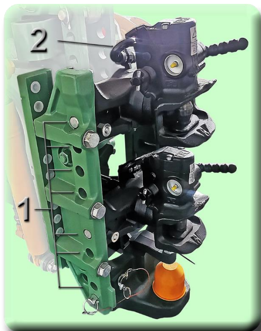
Komplettes, höhenverstellbares Anhängesystem.
